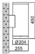
B: 上下照灯具尺寸图
